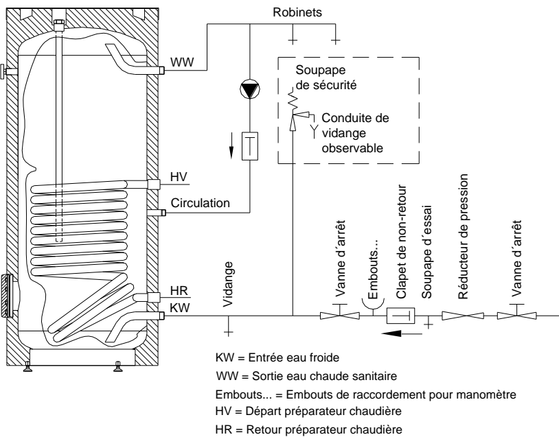
Schéma de raccordement (selon DIN 1988)
